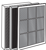
Předfiltr / True HEPA filtr ošetřený antimikrobiální vrstvou / uhlíkový CD filtr
